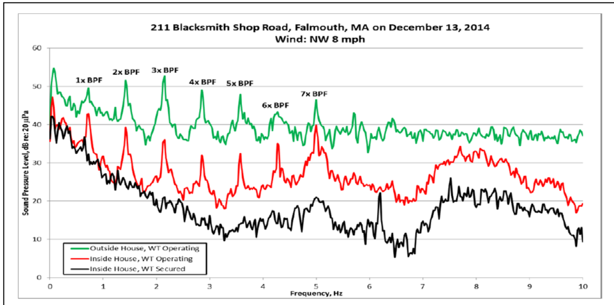
Bild 8: Frequenzanalyse eines tieffrequenten Schallsignales einer Windkraftanlage
